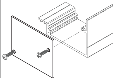
Πλαϊνή Τάπα του TV 80614 Side Cover For TV 80614
