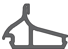
Κεντρικό Λάστιχο Περιστρεφόμενου Central Gasket for Pivot Window
