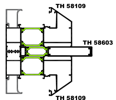
Τομή 13 Section 13
