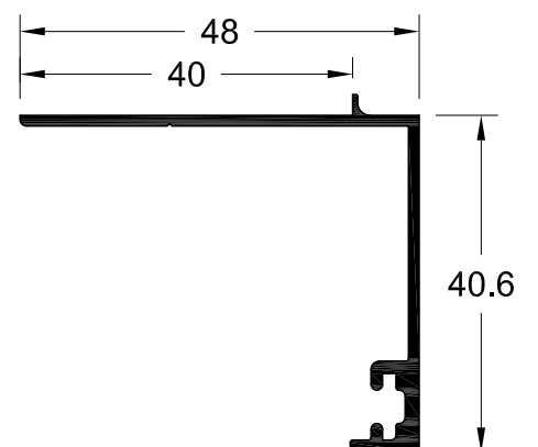
TV5 202 ΊΣΙΟ ΑΡΜΟΚΑΛΥΠΤΡΟ 394 gr/m STRAIGHT WALL-JOINING PROFILE
