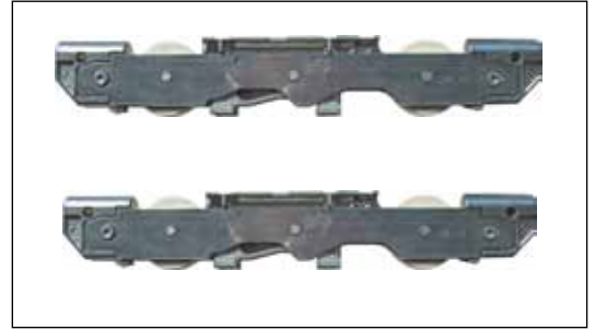
HS 400 HAUTAU - ΕΞΤΡΑ ΡΑΟΥΛΑ ΓΙΑ ΒΑΡΟΣ 400kg HS 400 HAUTAU - EXTRA ROLLERS FOR 400kg WEIGHT
