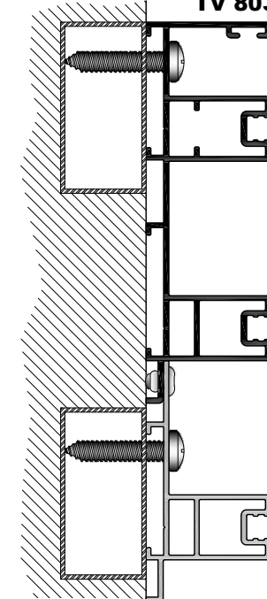
Ψευδόκασα Metal frame 20x40
