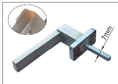
1325 CW/350 ΠΟΜΟΛΟ Europa LEVER HANDLE Europa
