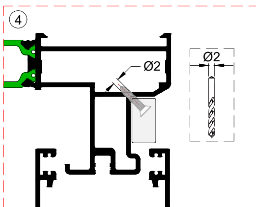
E2450-853 End cover for interlocking profiles Τάπα γάντζων επαλληλίων
