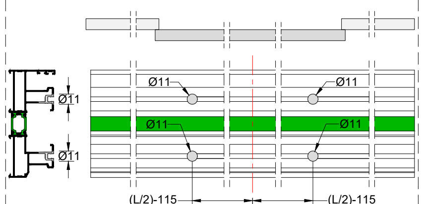
Holes for lower base Τρύπημα για κάτω βάσεις
