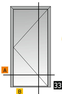
Single leaf door inward opening without threshold Μονόφυλλη πόρτα ανοιγόμενη μέσα με λάστιχο χωρίς κατωκάσι
