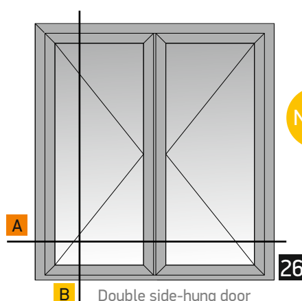
Double side-hung door inward opening without threshold Δίφυλλη πόρτα ανοιγόμενη μέσα με λάστιχο χωρίς κατωκάσι
