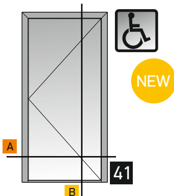
Single side- hung casement inward opening, hidden sash with threshold Μονόφυλλο ανοιγόμενο μέσα , κρυφό φύλλο με χαμηλό κατωκάσι
