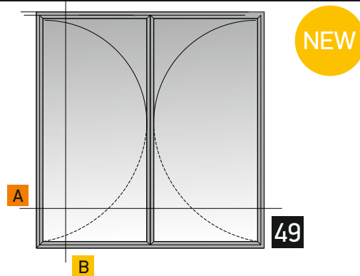
Double side-hung door, aller retour Δίφυλλη πόρτα διπλής κατεύθυνσης
