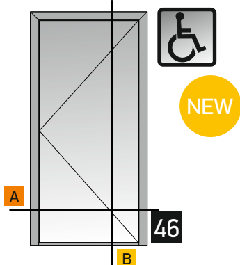
Single leaf door inward opening, hidden sash with threshold Μονόφυλλη πόρτα ανοιγόμενη μέσα, κρυφό φύλλο με χαμηλό κατωκάσι
