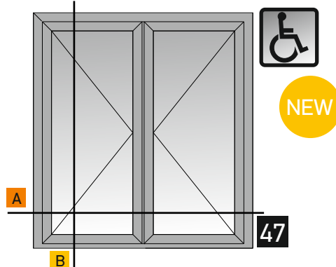
Double leaf door inward opening, hidden sash with threshold Δίφυλλη πόρτα ανοιγόμενη μέσα, κρυφό φύλλο με χαμηλό κατωκάσι
