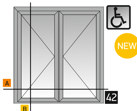
Double side- hung casement inward opening, hidden sash with threshold Δίφυλλο ανοιγόμενο μέσα , κρυφό φύλλο με χαμηλό κατωκάσι
