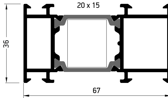
313-20-015-00 20 x 15
