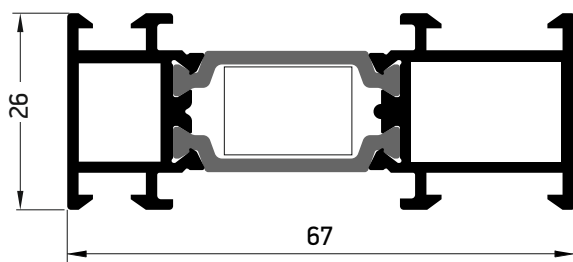
313-15-010-00 15 X 10
