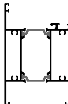
ΚΑΤΕΡΓΑΖΟΜΕΝΕΣ ΔΙΑΤΟΜΕΣ ΠΡΟΦΙΛ MILLING PROFILE
