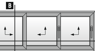
Τρίφυλλο επάλληλο ανασυρόμενο ΔΕΞΙ Triple sash parallel lift & slide RIGHT
