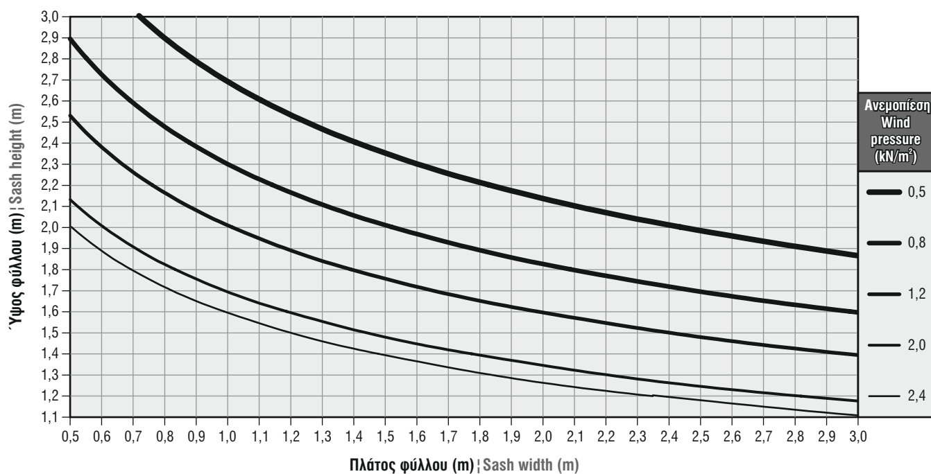
Μέγιστες διαστάσεις φύλλου για συγκεκριμένη ανεμοπίεση | Maximum sash dimensions for given wind pressure Φύλλα S366 & S356 - Άγκιστρο S363 | S366 & S356 sash profiles - S363 hook profile
