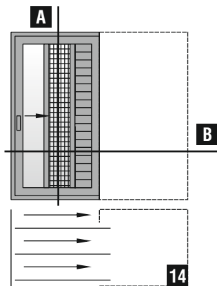
Μονόφυλλο χωνευτό συρόμενο με σήτα (φύλλο σήτας M868 ) και παντζούρι S325 One sash pocket sliding with fly-screen (M868 fly-screen sash) and shutter S325
