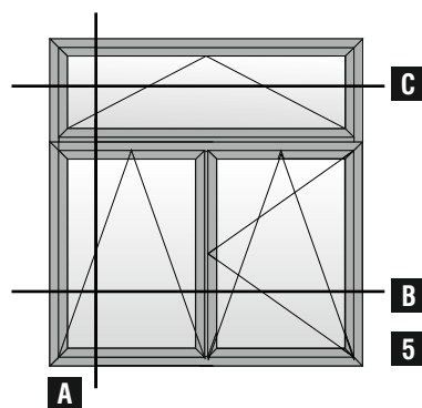
Δίφυλλο ανοιγόμενο - ανακλινόμενο παράθυρο με σταθερό επάνω Double Sash tilt & turn window with tilt on top
