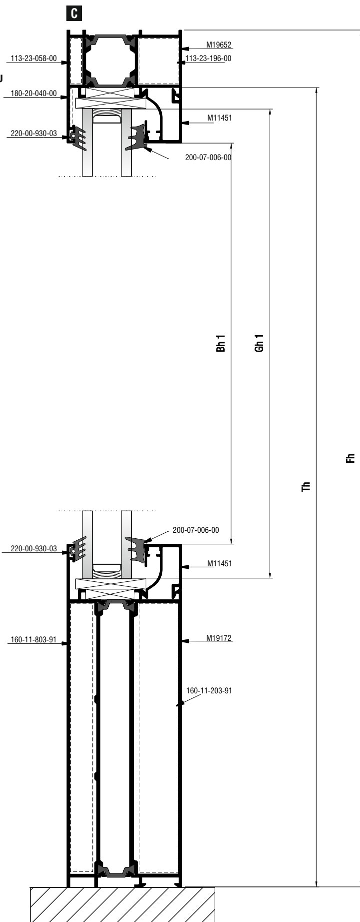
Πόρτες εισόδου Entrance doors
