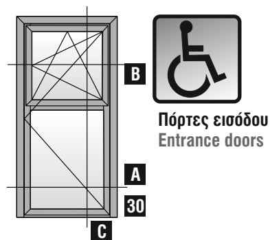
Μονόφυλλη πόρτα ανοιγόμενη μέσα με ενσωματωμένο παράθυρο Single leaf door inward opening with integrated window
