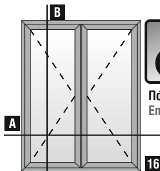
Δίφυλλη πόρτα εισόδου ανοιγόμενη έξω Double side-hung opening outward entrance door
