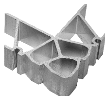
Γωνία σύνδεσης με διπλό χτύπημα 38,9x42mm | Double crimp corner cleat 38,9x42mm
