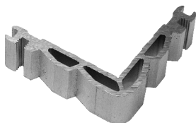
Γωνία σύνδεσης με διπλό χτύπημα Double crimp corner cleat
