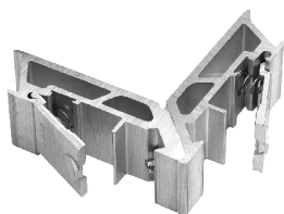
Γωνία σύνδεσης μηχανική Mechanical corner cleat
