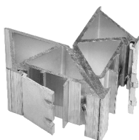
Γωνία σύνδεσης μηχανική 38,9x42mm Mechanical corner cleat 38,9x42mm
