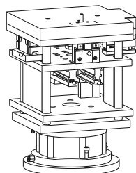
Πρέσα αέρος | Pneumatic punch press
