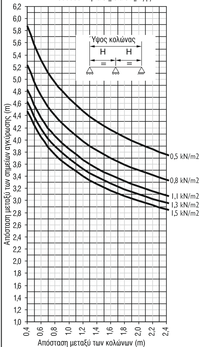
Πίνακας 5.8 M500009 - Τρία σημεία στήριξης
