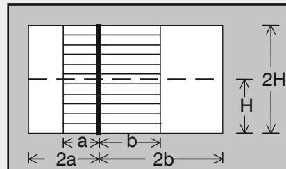
Πίνακας 2 Απαιτούμενη ροπή αδράνειας I_x για ομοιόμορφο φορτίο με τρία σημεία στήριξης Όριο ελαστικότητας = 7000kN / cm 4 Μέγιστο βέλος κάμψης f_{max}=l / 200 ή \leq 15mm
