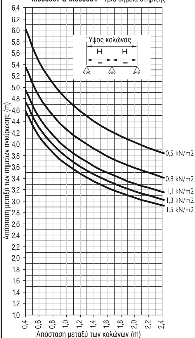
Πίνακας 5.18 M500007 & M500084 - Τρία σημεία στήριξης
