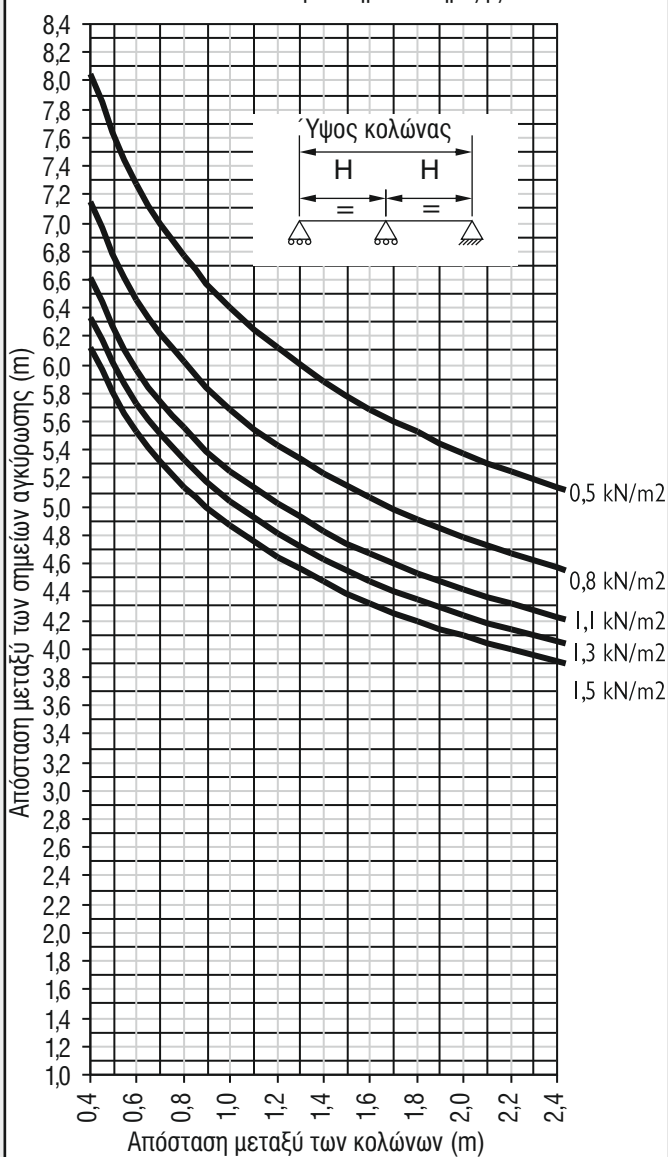
Πίνακας 5.12 M500013 - Τρία σημεία στήριξης
