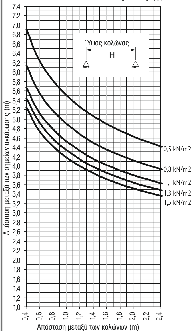
Πίνακας 5.21 M500011 & M500064 - Δύο σημεία στήριξης
