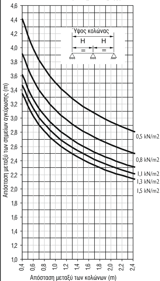
Πίνακας 5.4 M500005 - Τρία σημεία στήριξης
