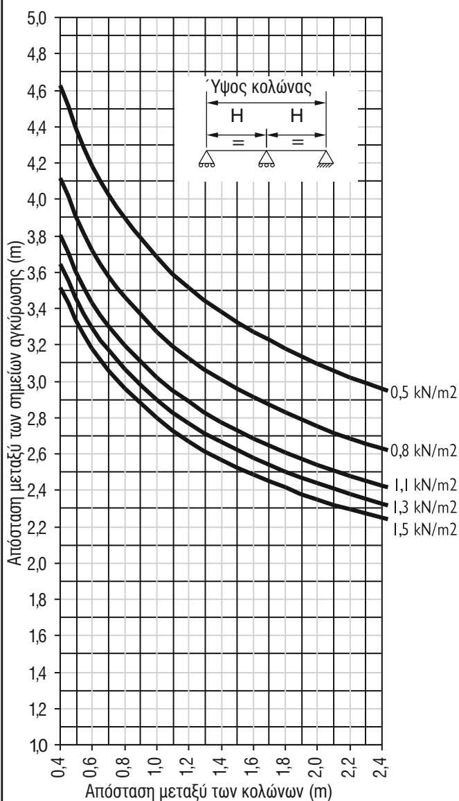
Πίνακας 5.16 M500005 & 40x40x2 - Τρία σημεία στήριξης
