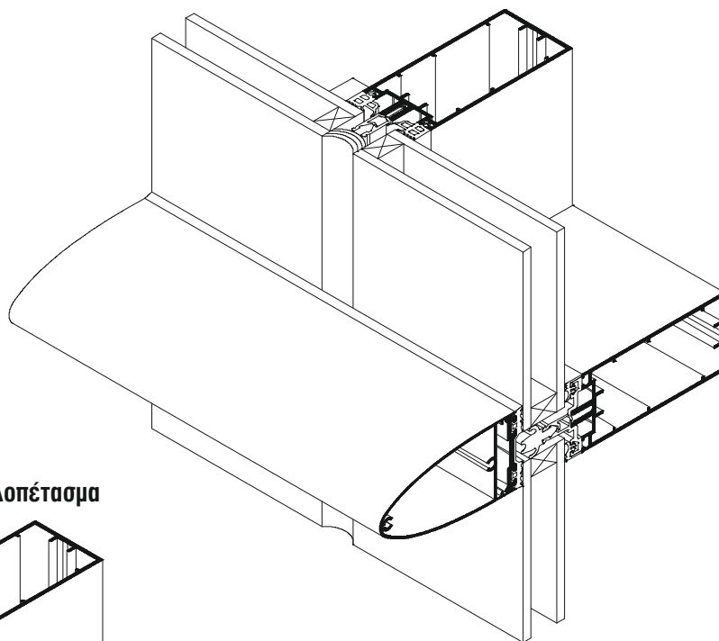
“Linear” υαλοπέτασμα
