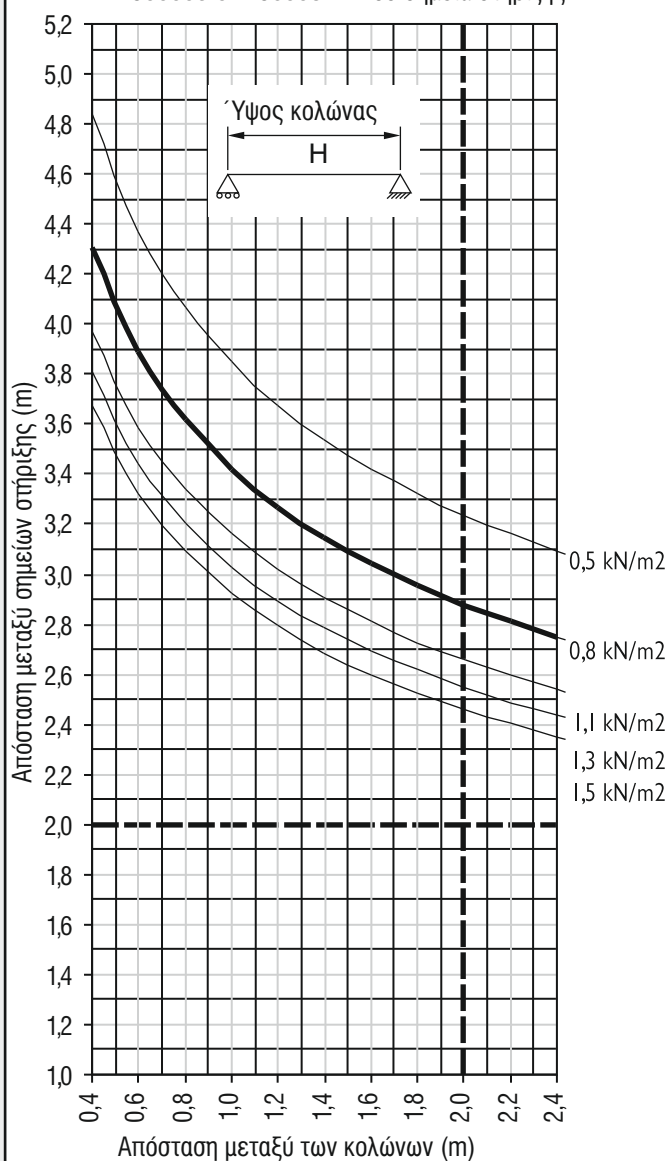
Πίνακας 5.17 M500009 & M500084 - Δύο σημεία στήριξης
