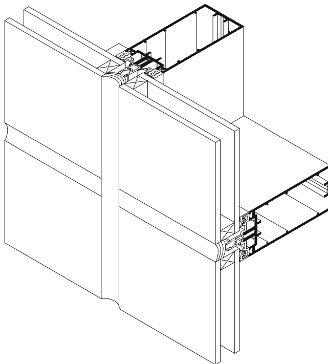
“Structural” υαλοπέτασμα
