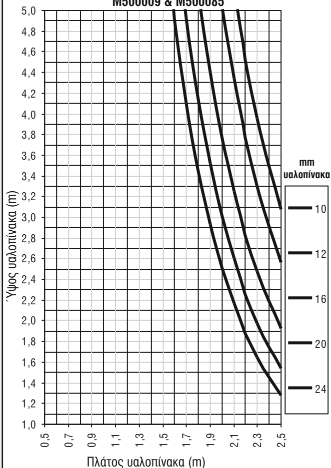
Πίνακας 6.8 M500009 & M500085
