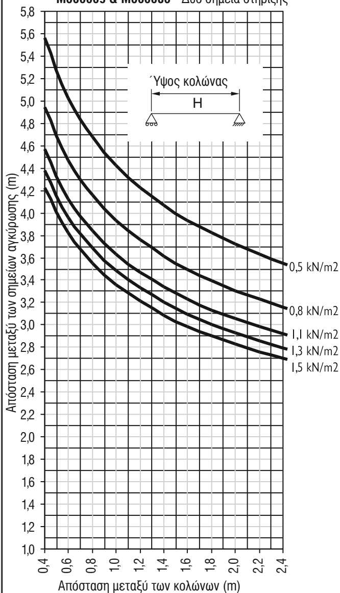
Πίνακας 5.19 M500009 & M500085 - Δύο σημεία στήριξης
