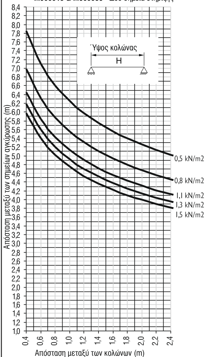
Πίνακας 5.23 M500013 & M500086 - Δύο σημεία στήριξης
