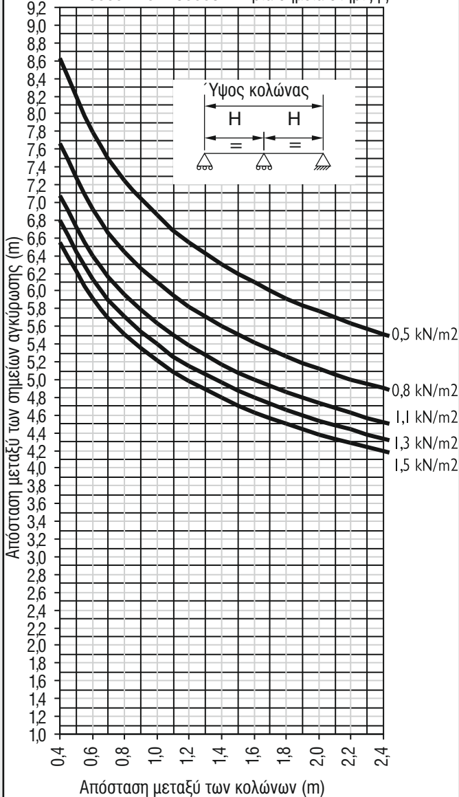
Πίνακας 5.22 M500011 & M500064 - Τρία σημεία στήριξης
