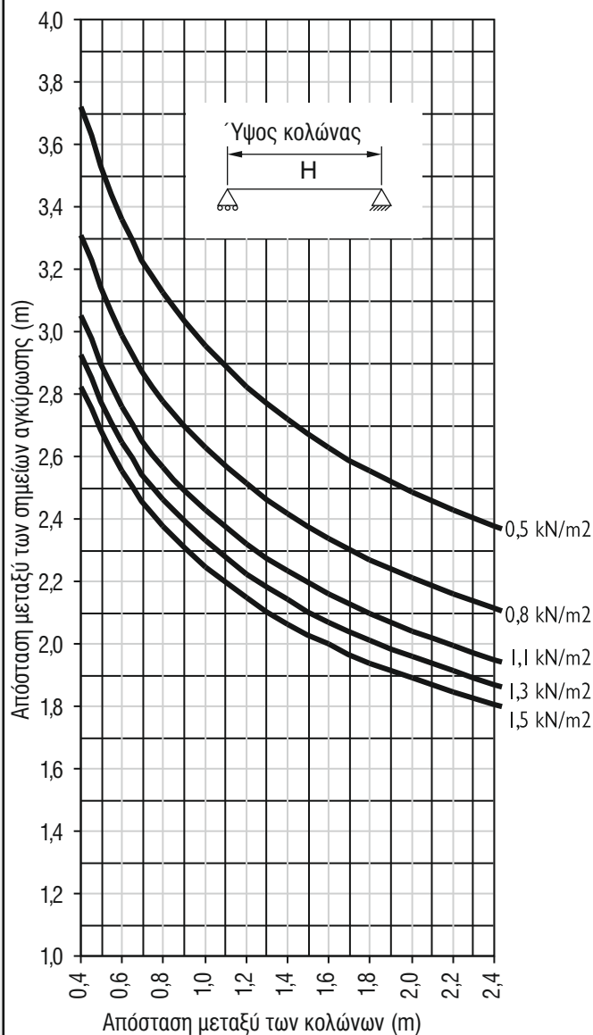
Πίνακας 5.15 M500005 & 40x40x2 - Δύο σημεία στήριξης
