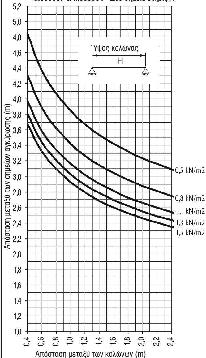
Πίνακας 5.17 M500007 & M500084 - Δύο σημεία στήριξης
