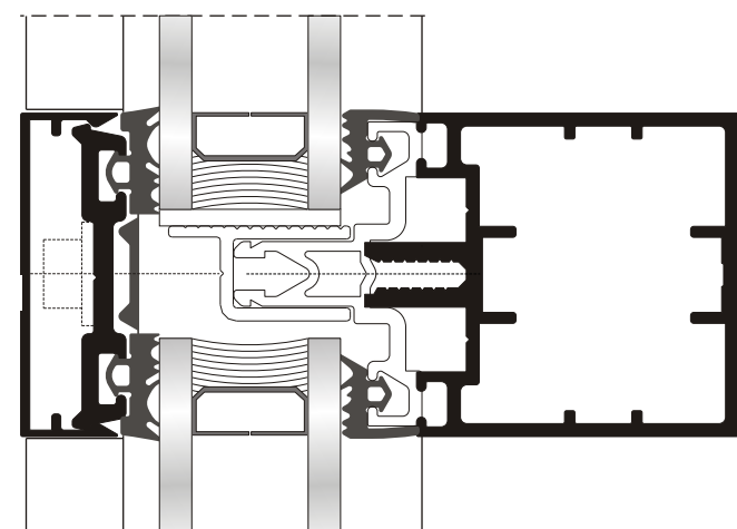
Εικόνα 5 Λεπτομέρειες τοποθέτησης υαλοπίνακα.
