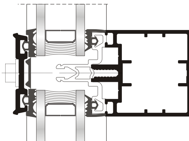
Εικόνα 6 Τα στηρίγματα των υαλοπινάκων μπορεί να αποτελούνται από τις πλάκες πίεσης και τα λάστιχα.
