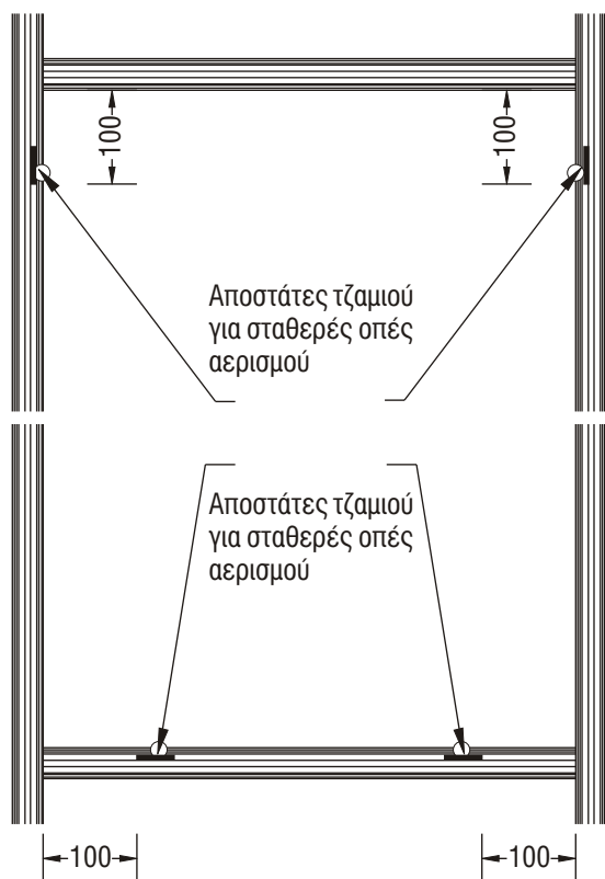
Εικόνα 3 Προσδιορισμός θέσης των τζαμιών.
