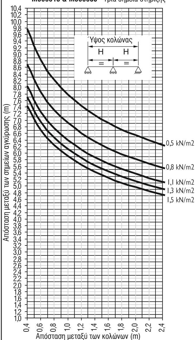
Πίνακας 5.24 M500013 & M500086 - Τρία σημεία στήριξης
