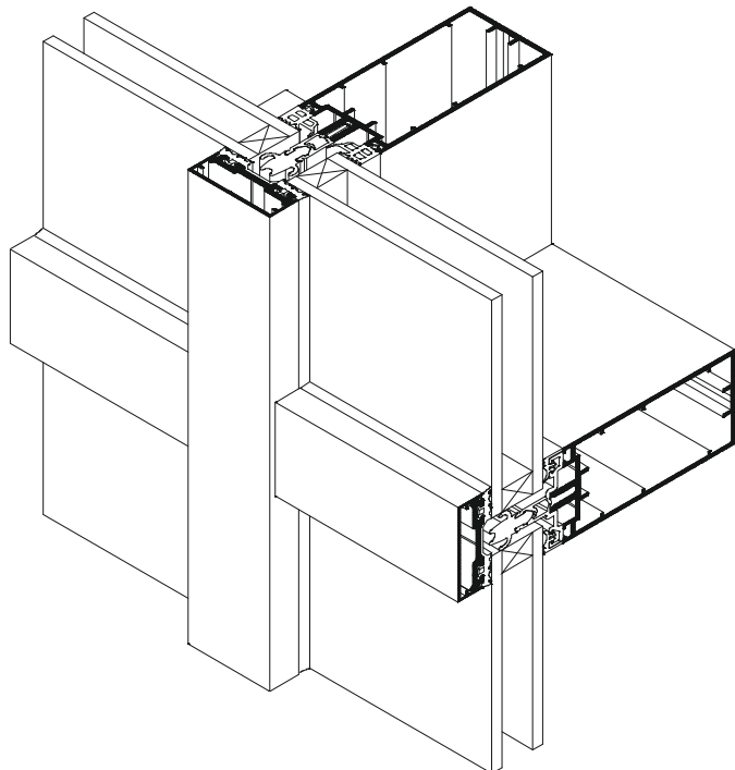
“Standard” υαλοπέτασμα
