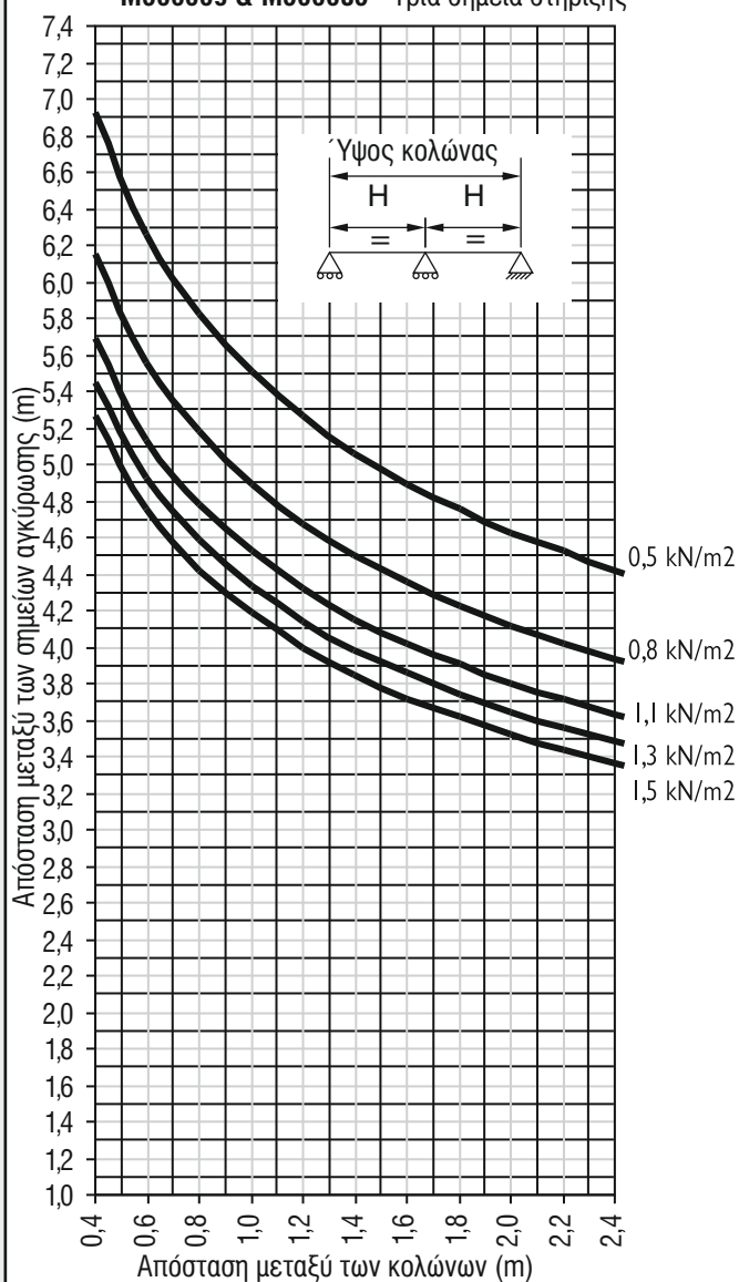
Πίνακας 5.20 M500009 & M500085 - Τρία σημεία στήριξης
