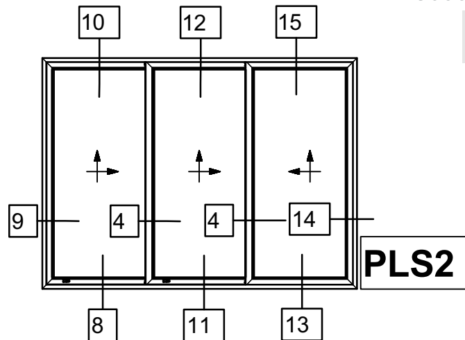
Three Sash Parallel Lift & Slide Window Τρίφυλλο Επάλληλο Ανασπώμενο
