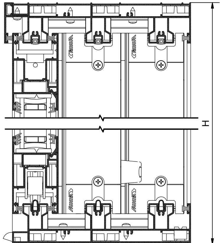
Three Sash Parallel Sliding Window with Narrow Interlock Τρίφυλλο Επάλληλο Συρόμενο με Στενό Γάντζο
