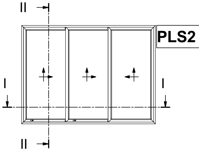
Three Sash Parallel Lift & Slide Window Τρίφυλλο Επάλληλο Ανασυρόμενο
