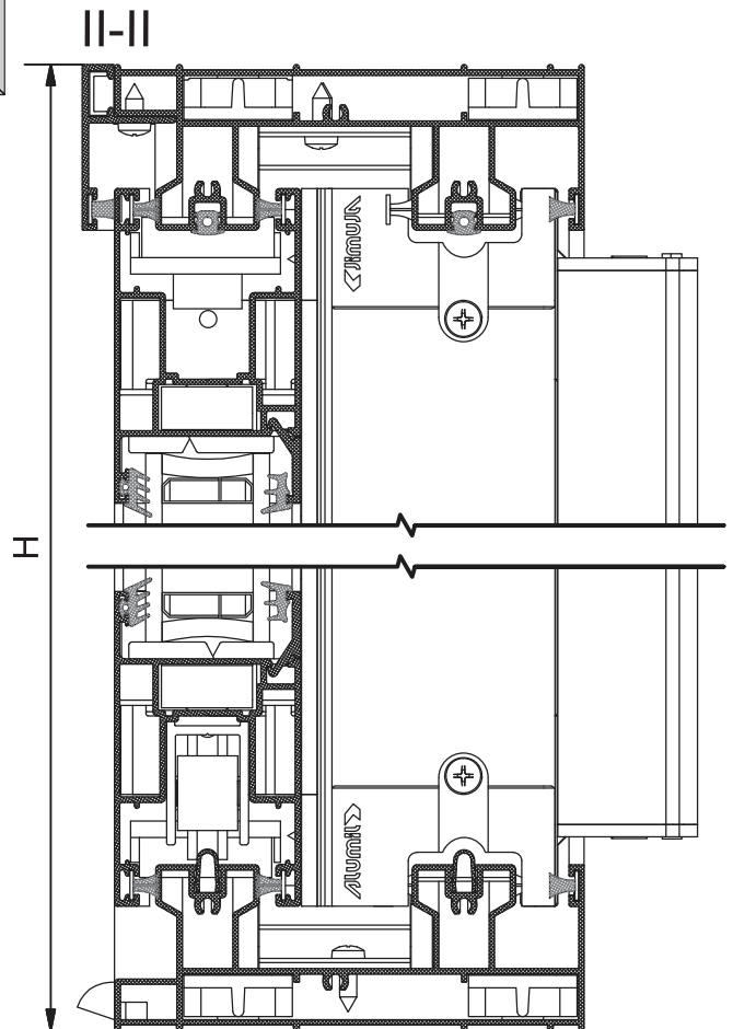
Four Sash Parallel with Meeting Stile Sliding Window Τετράφυλλο Φιλητό Επάλληλο Συρόμενο
