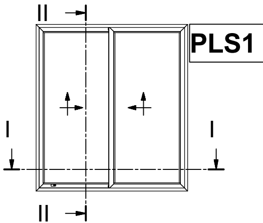
Two Sash Parallel Lift & Slide Window Δίφυλλο Επάλληλο Ανασυσρόμενο
