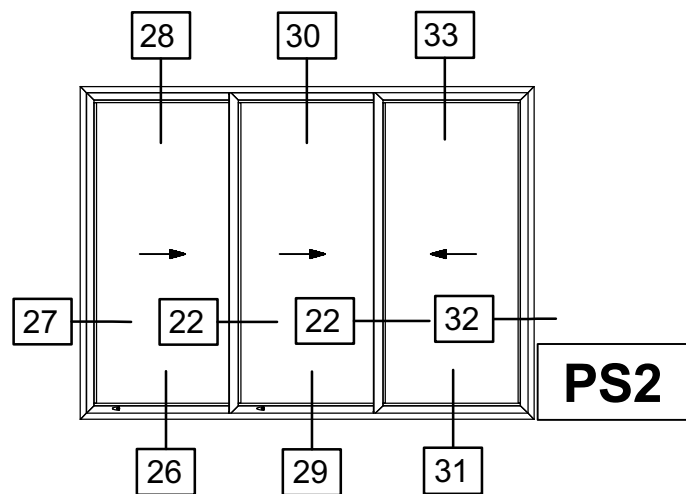
Three Sash Parallel Sliding Window Τρίφυλλο Επάλληλο Συρόμενο
