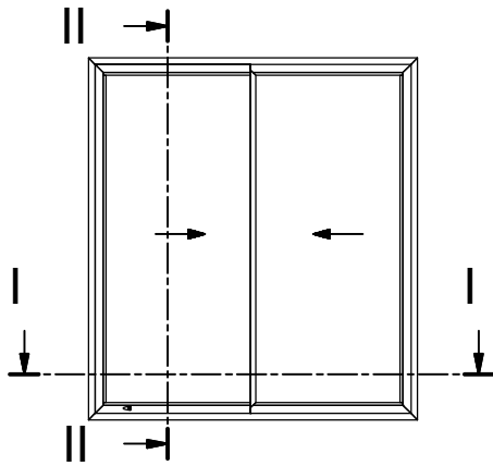
Two Sash Parallel Sliding Window with Narrow Interlock Δίφυλλο Επάλληλο Συρόμενο με Στενό Γάντζο
