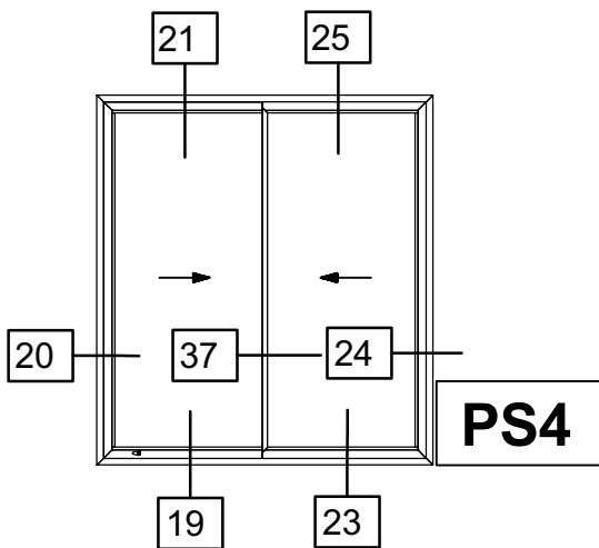
Two Sash Parallel Sliding Window with Narrow Interlock Δίφυλλο Επάλληλο Συρόμενο με Στενό Γάντζο
