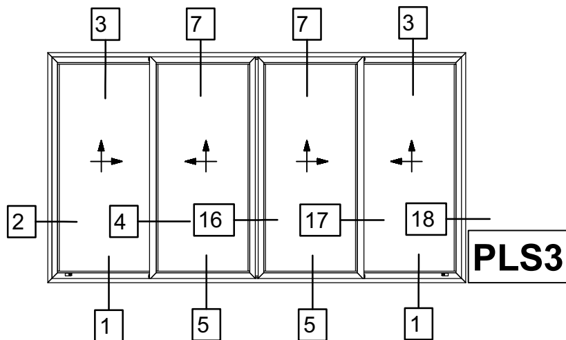
Four Sash Parallel with Meeting Stile Lift & Slide Window Τετράφυλλο Φιλητό Επάλληλο Ανασπώμενο
