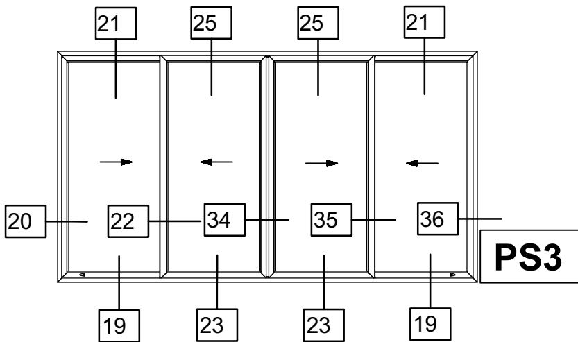
Four Sash Parallel with Meeting Stile Sliding Window Τετράφυλλο Φιλητό Επάλληλο Συρόμενο
