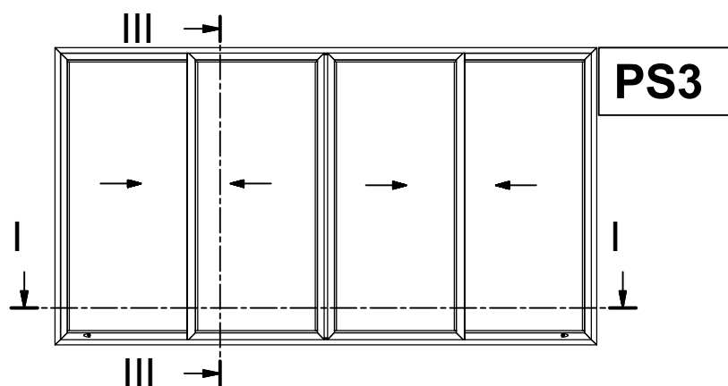
Four Sash Parallel with Meeting Stile Sliding Window Τετράφυλλο Φιλητό Επάλληλο Συρόμενο
