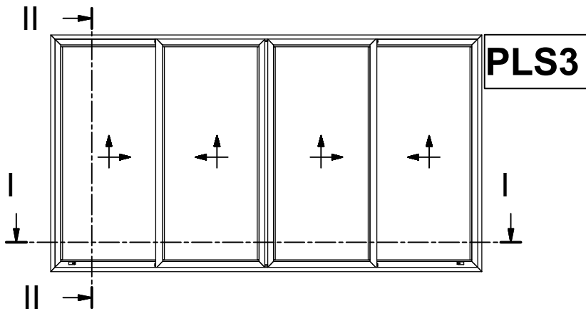
Four Sash Parallel with Meeting Stile Lift & Slide Window Τετράφυλλο Φιλητό Επάλληλο Ανασυρόμενο
