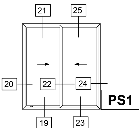
Two Sash Parallel Sliding Window Δίφυλλο Επάλληλο Συρόμενο
