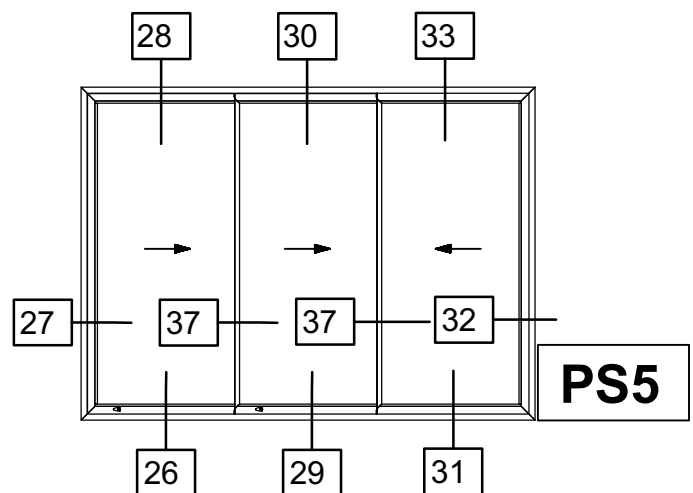
Three Sash Parallel Sliding Window with Narrow Interlock Τρίφυλλο Επάλληλο Συρόμενο με Στενό Γάντζο
