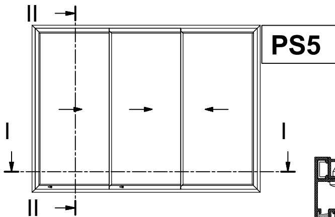
Three Sash Parallel Sliding Window with Narrow Interlock Τρίφυλλο Επάλληλο Συρόμενο με Στενό Γάντζο
