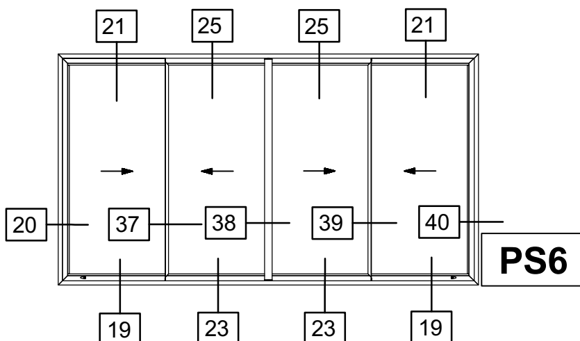
Four Sash Parallel with Meeting Stile Sliding Window Τετράφυλλο Φιλητό Επάλληλο Συρόμενο
