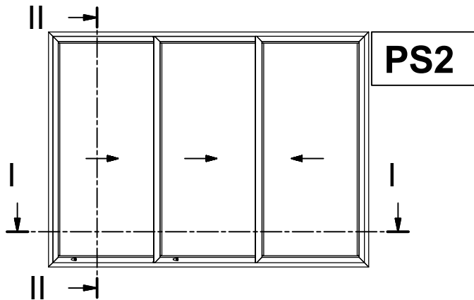
Three Sash Parallel Sliding Window Τρίφυλλο Επάλληλο Συρόμενο
