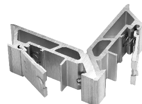
Γωνία σύνδεσης κουμπωτή | Spring cleat
