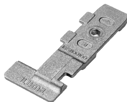
Σύνδεσμος ταν χυτός έξω (δεξιά) Outer cast transom-mullion cleat (right)
