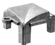
Χυτή γωνία για πηχάκι M11462 Cast corner for M11462 glazing bead
