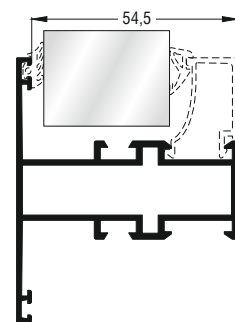
Για ταυ | For transom-mullion M15065
