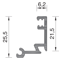
101-081 ΒΑΡΟΣ WEIGHT 251 GR/M
