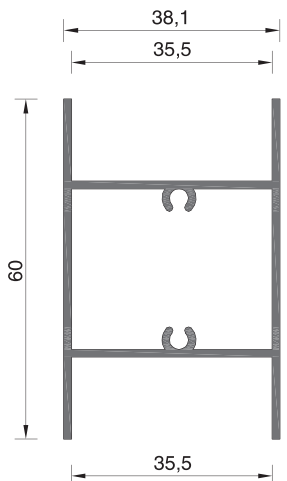
101-029 ΒΑΡΟΣ WEIGHT 730 GR/M
