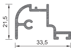
108-055 ΒΑΡΟΣ WEIGHT 356 GR/M
