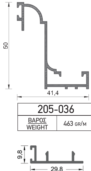
205-036 ΒΑΡΟΣ WEIGHT 463 GR/M
