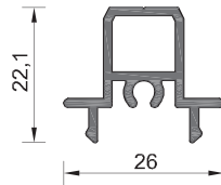
210-013 ΒΑΡΟΣ WEIGHT 303 GR/M
