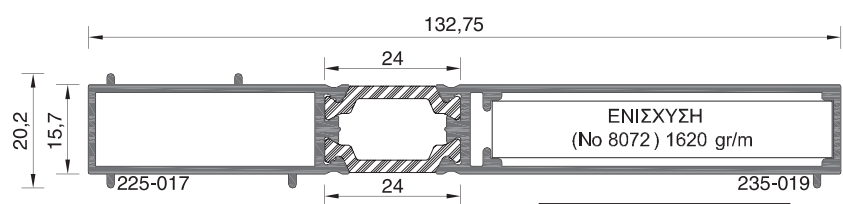
225-29 ΒΑΡΟΣ WEIGHT 1355 GR/M
