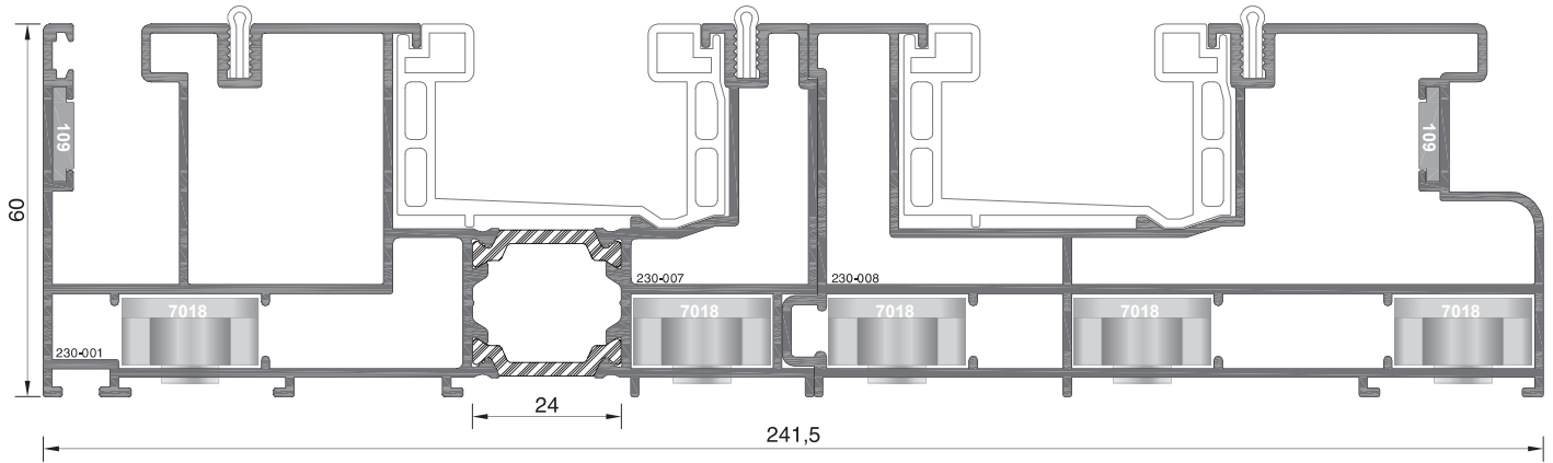
ΤΡΙΠΛΟΣ ΟΔΗΓΟΣ (ΕΣΩΤΕΡΙΚΟ ΠΡΟΦΙΛ) TRIPLE FRAME (INNER PROFILE)
