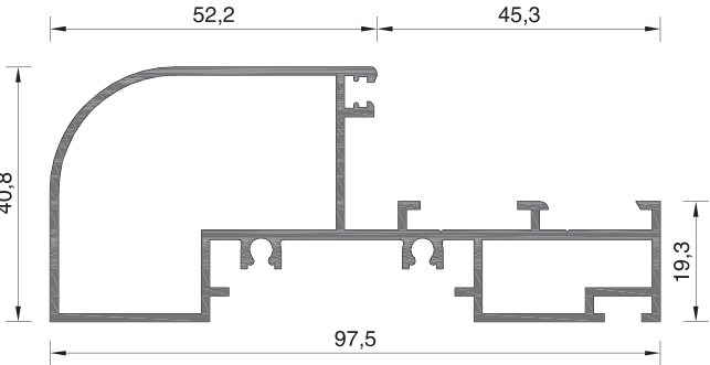
215-006 ΒΑΡΟΣ WEIGHT 1219 GR/M
