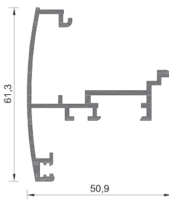
108-013 ΒΑΡΟΣ WEIGHT 710 GR/M
