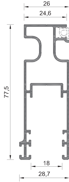
225-026 ΒΑΡΟΣ WEIGHT 929 GR/M
