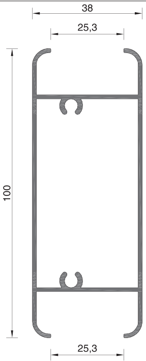
101-152 ΒΑΡΟΣ WEIGHT 1096 GR/M
