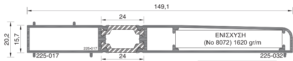
225-32 ΒΑΡΟΣ WEIGHT 1468 GR/M
