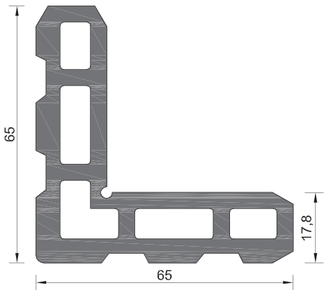
101-071 ΒΑΡΟΣ WEIGHT 3208 GR/M
