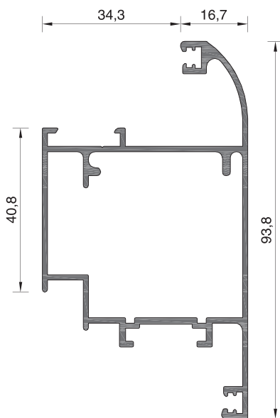
108-069 ΒΑΡΟΣ WEIGHT 1199 GR/M
