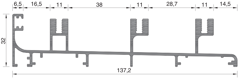
220-005 ΒΑΡΟΣ WEIGHT 1736 GR/M
