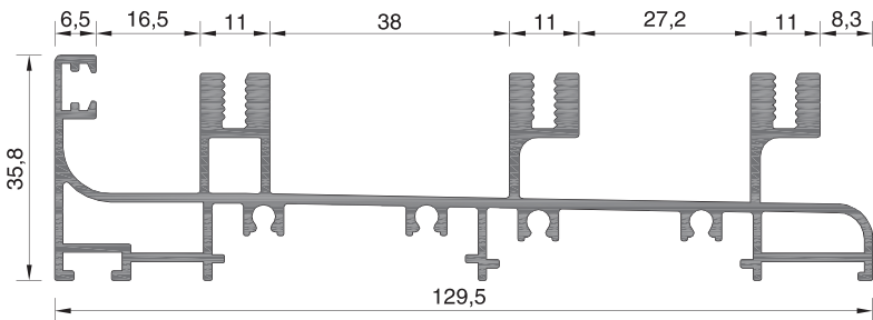
220-009 ΒΑΡΟΣ WEIGHT 1993 GR/M
