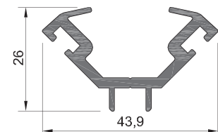
130-50-305 ΒΑΡΟΣ WEIGHT 574 GR/M
