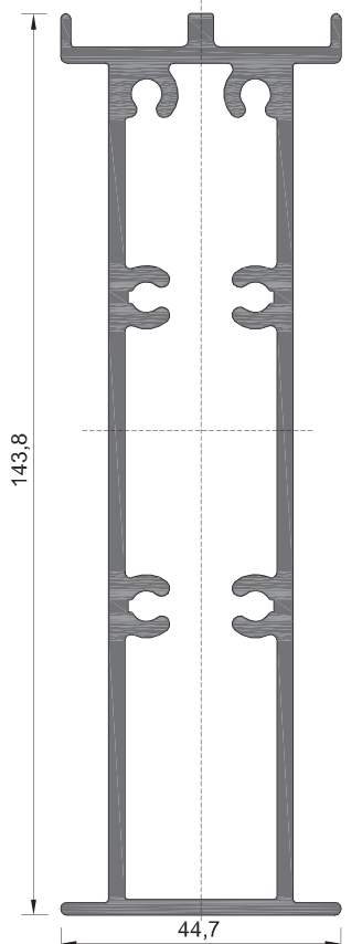
130-50-404 ΒΑΡΟΣ WEIGHT 3156 GR/M
