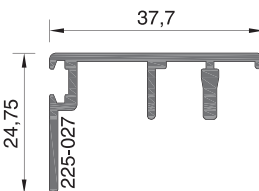
225-027 ΒΑΡΟΣ WEIGHT 367 GR/M
