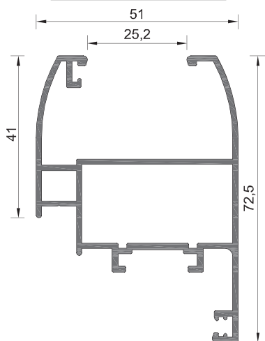
108-045 ΒΑΡΟΣ WEIGHT 1045 GR/M
