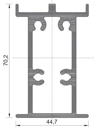
130-50-402 ΒΑΡΟΣ WEIGHT 1944 GR/M
