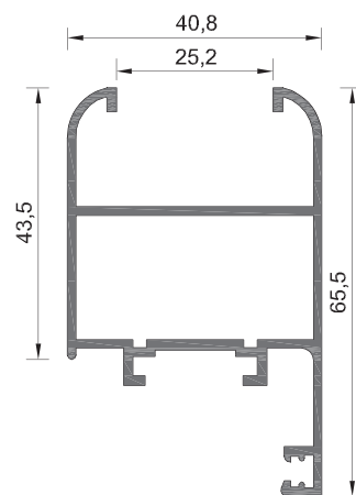
108-009 ΒΑΡΟΣ WEIGHT 829 GR/M
