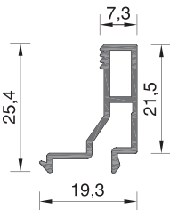
108-026B ΒΑΡΟΣ WEIGHT 225 GR/M
