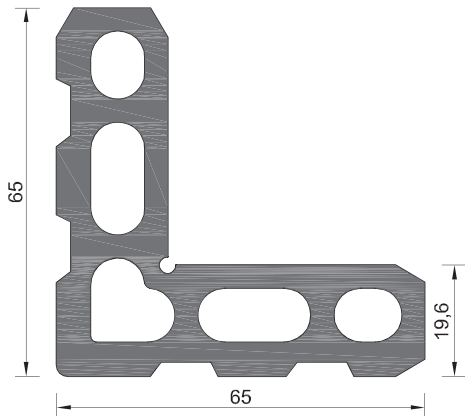
101-075 ΒΑΡΟΣ WEIGHT 3541 GR/M
