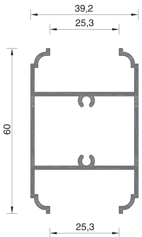
101-028 ΒΑΡΟΣ WEIGHT 795 GR/M
