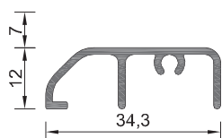
108-056 ΒΑΡΟΣ WEIGHT 258 GR/M
