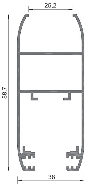
215-007 ΒΑΡΟΣ WEIGHT 1150 GR/M
