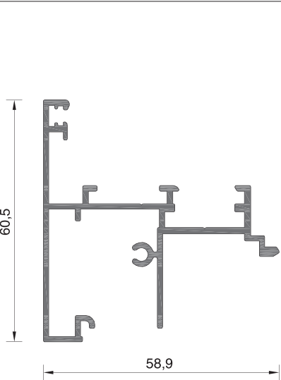
101-035B ΒΑΡΟΣ WEIGHT 861 GR/M
