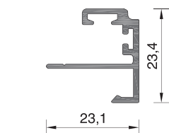
225-019 ΒΑΡΟΣ WEIGHT 257 GR/M
