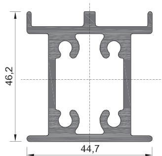
130-50-401 ΒΑΡΟΣ WEIGHT 1636 GR/M
