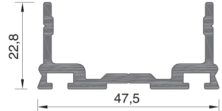
130-50-318 ΒΑΡΟΣ WEIGHT 626 GR/M
