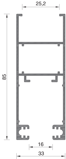
225-046 ΒΑΡΟΣ WEIGHT 1085 GR/M
