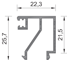
108-027 ΒΑΡΟΣ WEIGHT 304 GR/M
