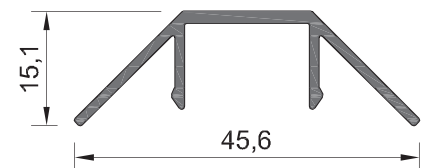
130-50-306 ΒΑΡΟΣ WEIGHT 269 GR/M
