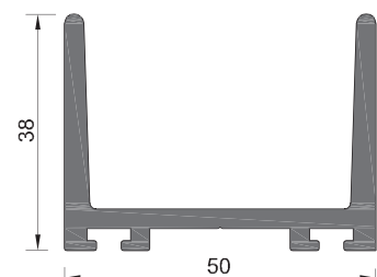
130-50-304 ΒΑΡΟΣ WEIGHT 1151 GR/M
