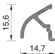
108-057A ΒΑΡΟΣ WEIGHT 126 GR/M
