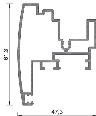
108-070 ΒΑΡΟΣ WEIGHT 992 GR/M
