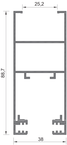
215-008 ΒΑΡΟΣ WEIGHT 1204 GR/M
