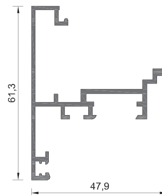
108-012 ΒΑΡΟΣ WEIGHT 685 GR/M
