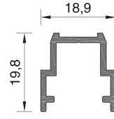
215-022 ΒΑΡΟΣ WEIGHT 219 GR/M
