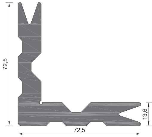
109-031 ΒΑΡΟΣ WEIGHT 3803 GR/M
