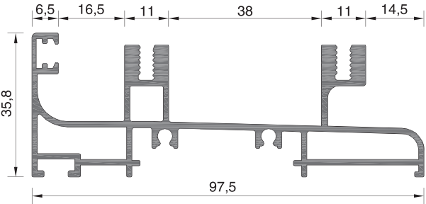
220-006 ΒΑΡΟΣ WEIGHT 1495 GR/M
