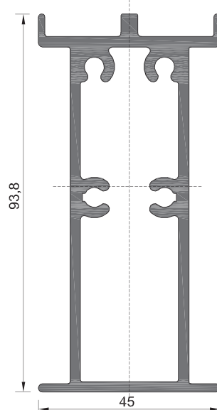
130-50-403 ΒΑΡΟΣ WEIGHT 2268 GR/M
