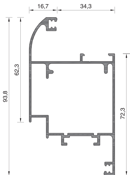
108-068 ΒΑΡΟΣ WEIGHT 1199 GR/M
