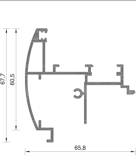
101-034C ΒΑΡΟΣ WEIGHT 1005 GR/M
