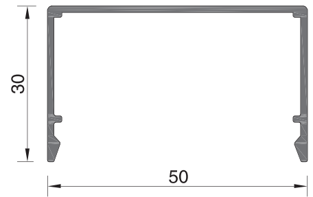
130-50-319 ΒΑΡΟΣ WEIGHT 383 GR/M
