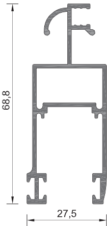
215-013 ΒΑΡΟΣ WEIGHT 816 GR/M
