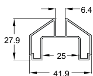
Code/Κωδικός 994-914 Weight/Βάρος 489 gr/m Length/Μήκος 6 m
