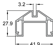
Code/Κωδικός 992-904 Weight/Βάρος 651 gr/m Length/Μήκος 6 m
