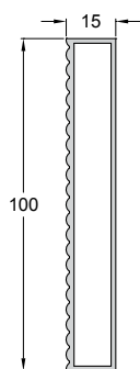
Code/Κωδικός 070-005 Weight/Βάρος 1005 gr/m Length/Μήκος 6 m
