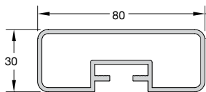
Code/Κωδικός F50-201 Weight / Βάρος 1.350 kg/m Length/Μήκος 6 m
