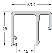
Code/Κωδικός | FSN-301 Weight / Βάρος | 607 gr/m Length/Μήκος | 6 m
