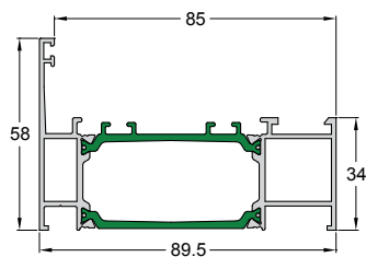
Code/Κωδικός 4900-101 Weight/Βάρος 1429 gr/m Length/Μήκος 6 m Pack/Δέμα 2 Bars/Βέργες
