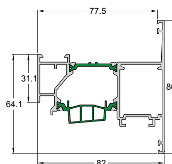
Code/Κωδικός 4750-227 Weight/Βάρος 1704 gr/m Length/Μήκος 6 m Pack/Δέμα 2 Bars/Βέργες
