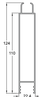
Code/Κωδικός PAT99-045 Weight/Βάρος 1046 gr/m Length/Μήκος 6 m Pack/Δέμα 5 Bars/Βέργες
