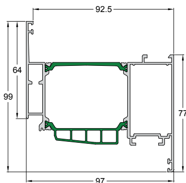
Code/Κωδικός 4900-202 Weight/Βάρος 2005 gr/m Length/Μήκος 6 m Pack/Δέμα 1 Bar/Βέργα
