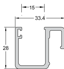
Code/Κωδικός | FSN-300 Weight / Βάρος | 607 gr/m Length/Μήκος | 6 m
