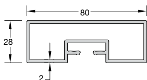
Code/Κωδικός CLS-202 Weight / Βάρος 1360 gr/m Length/Μήκος 6 m
