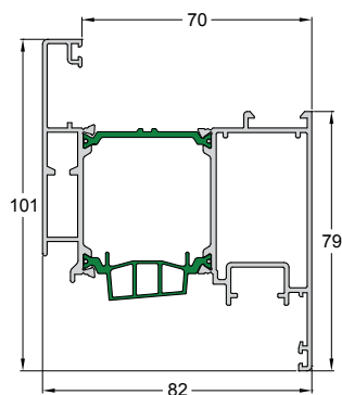
Code/Κωδικός 4750-217 Weight/Βάρος 1926 gr/m Length/Μήκος 6.5 m Pack/Δέμα 2 Bars/Βέργες
