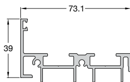
Code/Κωδικός 994-504 Weight/Βάρος 1104 gr/m Length/Μήκος 6 m
