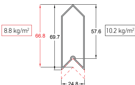
Code/Κωδικός 245-013 Weight/Βάρος 590 gr/m Length/Μήκος 6 m
