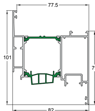
Code/Κωδικός 4750-233 Weight/Βάρος 1882 gr/m Length/Μήκος 6.5 m Pack/Δέμα 2 Bars/Βέργες
