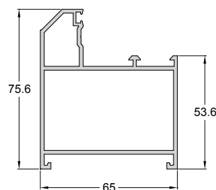
Code/Κωδικός 994-204 Weight/Βάρος 1495 gr/m Length/Μήκος 6 m
