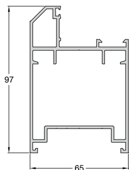
Code/Κωδικός 994-214 Weight/Βάρος 1972 gr/m Length/Μήκος 6 m
