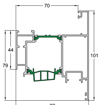
Code/Κωδικός 4750-218 Weight/Βάρος 1988 gr/m Length/Μήκος 6.5 m Pack/Δέμα 2 Bars/Βέργες
