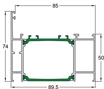
Code/Κωδικός 4900-102 Weight/Βάρος 1724 gr/m Length/Μήκος 6 m Pack/Δέμα 2 Bars/Βέργες
