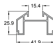
Code/Κωδικός 994-915 Weight/Βάρος 475 gr/m Length/Μήκος 6 m
