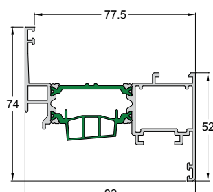
Code/Κωδικός 4750-221 Weight/Βάρος 1418 gr/m Length/Μήκος 6 m Pack/Δέμα 2 Bars/Βέργες
