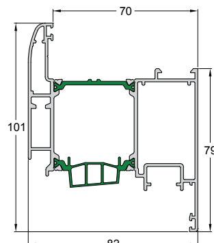
Code/Κωδικός 4750-234 Weight/Βάρος 1989 gr/m Length/Μήκος 6.5 m Pack/Δέμα 2 Bars/Βέργες
