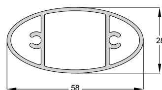
Code/Κωδικός | FSN-304 Weight / Βάρος | 804 gr/m Length/Μήκος | 6 m
