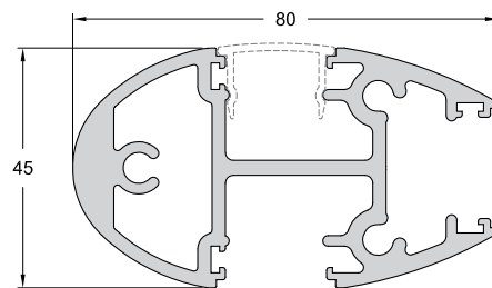
Code/Κωδικός FSN-102 Weight / Βάρος 2384 gr/m Length/Μήκος 6 m
