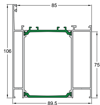
Code/Κωδικός 4900-103 Weight/Βάρος 2407 gr/m Length/Μήκος 6 m Pack/Δέμα 1 Bar/Βέργα
