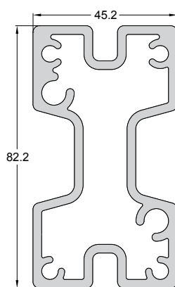
Code/Κωδικός 2200-903 Weight / Βάρος 2758 gr/m Length/Μήκος 6 m
