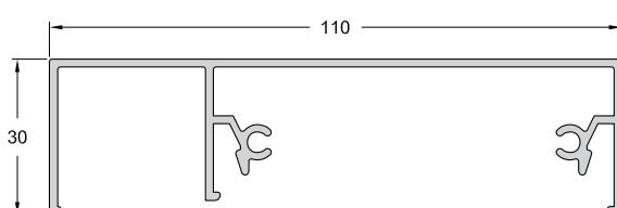
Code/Κωδικός | FSN-223 Weight / Βάρος | 1006 gr/m Length/Μήκος | 6 m
