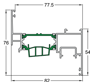
Code/Κωδικός 4750-231 Weight/Βάρος 1421 gr/m Length/Μήκος 6 m Pack/Δέμα 2 Bars/Βέργες
