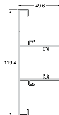
Code/Κωδικός 994-302 Weight/Βάρος 1815 gr/m Length/Μήκος 6 m
