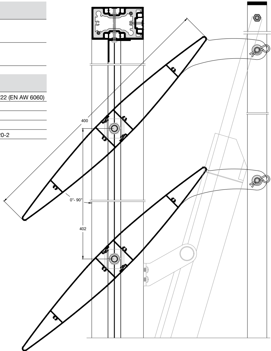
Elliptical design louver with adjustable incline Πτερύγιο ελλειπτικού σχεδιασμού ρυθμιζόμενης κλίσης
