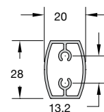
Code/Κωδικός CLS-304 Weight / Βάρος 389 gr/m Length/Μήκος 6 m
