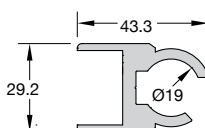
Code/Κωδικός CLS-904 Weight / Βάρος 1104 gr/m Length/Μήκος 6 m
