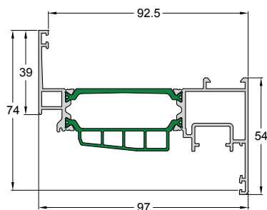
Code/Κωδικός 4900-215 Weight/Βάρος 1560 gr/m Length/Μήκος 6 m Pack/Δέμα 2 Bars/Βέργες
