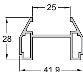
Code/Κωδικός 992-903 Weight/Βάρος 532 gr/m Length/Μήκος 6 m
