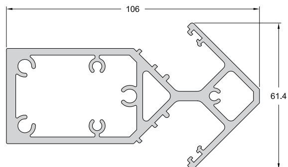
Code/Κωδικός FSN-104 Weight / Βάρος 3118 gr/m Length/Μήκος 6 m
