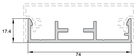
Code/Κωδικός FSN-201 Weight / Βάρος 872 gr/m Length/Μήκος 6 m
