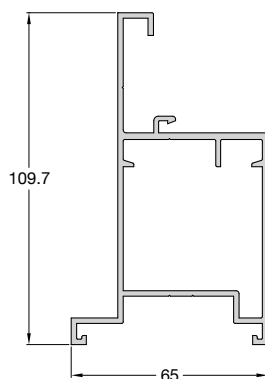
Code/Κωδικός 994-217 Weight/Βάρος 1723 gr/m Length/Μήκος 6 m
