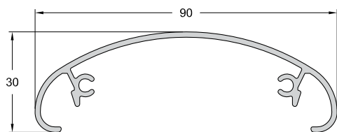
Code/Κωδικός | FSN-222 Weight / Βάρος | 736 gr/m Length/Μήκος | 6 m
