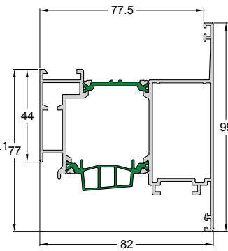
Code/Κωδικός 4750-228 Weight/Βάρος 1922 gr/m Length/Μήκος 6.5 m Pack/Δέμα 2 Bars/Βέργες
