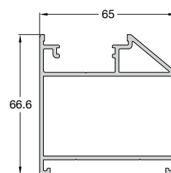
Code/Κωδικός 994-206 Weight/Βάρος 1517 gr/m Length/Μήκος 6 m
