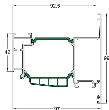
Code/Κωδικός 4900-217 Weight/Βάρος 2039 gr/m Length/Μήκος 6 m Pack/Δέμα 1 Bar/Βέργα
