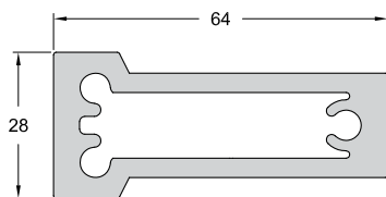
Code/Κωδικός FSN-101 Weight / Βάρος 1980 gr/m Length/Μήκος 6 m
