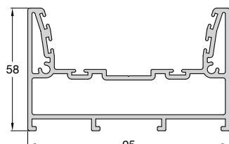
Code/Κωδικός 994-107 Weight/Βάρος 2372 gr/m Length/Μήκος 6 m
