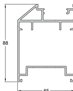
Code/Κωδικός 994-216 Weight/Βάρος 1987 gr/m Length/Μήκος 6 m
