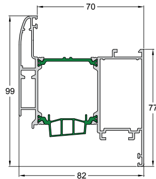
Code/Κωδικός 4750-224 Weight/Βάρος 1973 gr/m Length/Μήκος 6.5 m Pack/Δέμα 2 Bars/Βέργες
