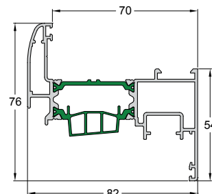
Code/Κωδικός 4750-235 Weight/Βάρος 1946 gr/m Length/Μήκος 6.5 m Pack/Δέμα 2 Bars/Βέργες
