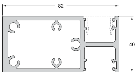
Code/Κωδικός FSN-103 Weight / Βάρος 2367 gr/m Length/Μήκος 6 m
