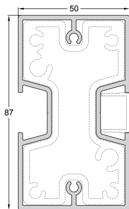
Code/Κωδικός 2200-102 Weight / Βάρος 1885 gr/m Length/Μήκος 6 m
