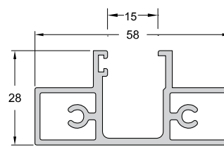
Code/Κωδικός | FSN-303 Weight / Βάρος | 976 gr/m Length/Μήκος | 6 m
