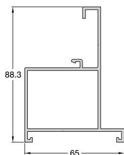
Code/Κωδικός 994-207 Weight/Βάρος 1353 gr/m Length/Μήκος 6 m
