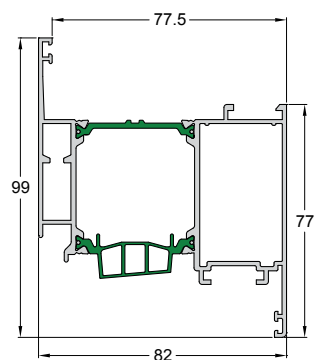
Code/Κωδικός 4750-223 Weight/Βάρος 1866 gr/m Length/Μήκος 6.5 m Pack/Δέμα 2 Bars/Βέργες
