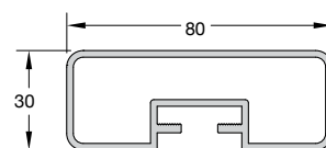
Code/Κωδικός F50-201 Weight / Βάρος 1350 gr/m Length/Μήκος 6 m
