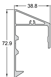
Code/Κωδικός 994-905 Weight/Βάρος 886 gr/m Length/Μήκος 6 m
