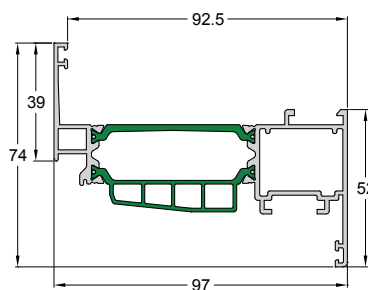
Code/Κωδικός 4900-201 Weight/Βάρος 1557 gr/m Length/Μήκος 6 m Pack/Δέμα 2 Bars/Βέργες
