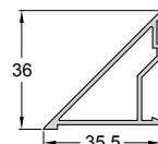
Code/Κωδικός 994-901 Weight/Βάρος 416 gr/m Length/Μήκος 6 m
