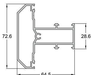
Code/Κωδικός 994-301 Weight/Βάρος 1484 gr/m Length/Μήκος 6 m
