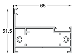
Code/Κωδικός 994-103 Weight/Βάρος 1295 gr/m Length/Μήκος 6 m
