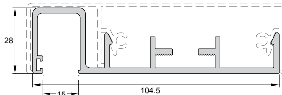
Code/Κωδικός FSN-203 Weight / Βάρος 1446 gr/m Length/Μήκος 6 m
