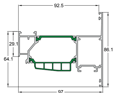
Code/Κωδικός 4900-203 Weight/Βάρος 1819 gr/m Length/Μήκος 6 m Pack/Δέμα 2 Bars/Βέργες
