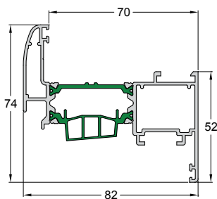
Code/Κωδικός 4750-229 Weight/Βάρος 1694 gr/m Length/Μήκος 6.5 m Pack/Δέμα 2 Bars/Βέργες
