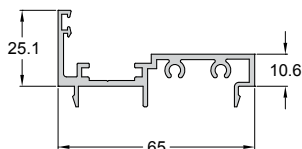
Code/Κωδικός 994-920 Weight/Βάρος 808 gr/m Length/Μήκος 6 m
