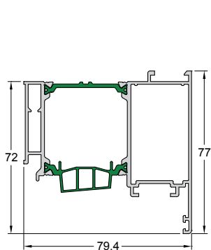
Code/Κωδικός 4750-229 Weight/Βάρος 1694 gr/m Length/Μήκος 6.5 m Pack/Δέμα 2 Bars/Βέργες
