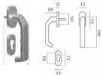
Μονή λαβή πόρτας σπαστή - Πείρος - Ροζέτα
