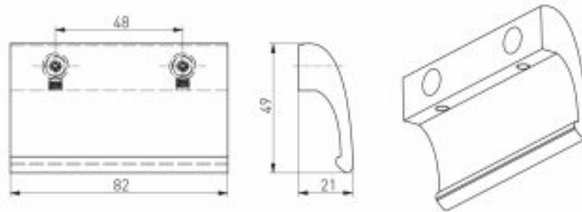
Συγκρατητής φύλλου euro groove
