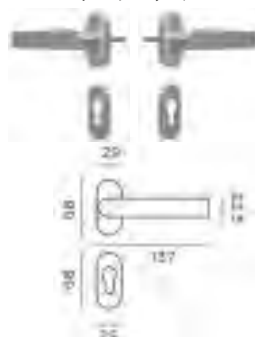
Μονή/Ζεύγος λαβής πόρτας με ενιαία πλάκα ροζέτας
