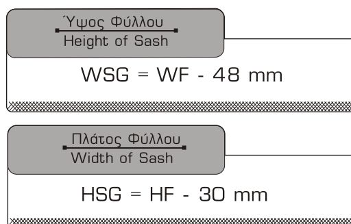
Κοπές Μονόφυλλου με φύλλο τελάρο και την χρήση του EL 5478
