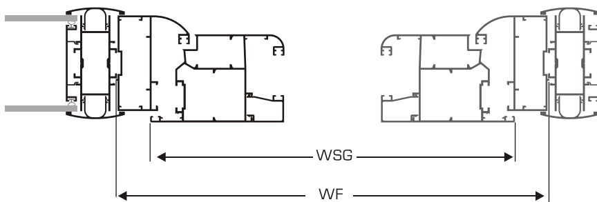
Κοπές Μονόφυλλου με την χρήση ταμπλά Single Sash Cuttings using bottom rail profile
