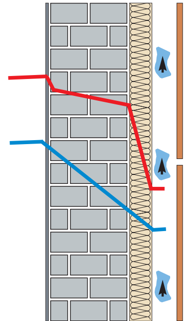
ΠΡΟΣΟΨΗ ΜΕ ΕΞΩΤΕΡΙΚΗ ΘΕΡΜΟΜΟΝΩΣΗ
