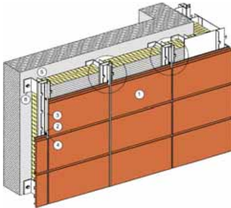
Κλειστός αρμός 9mm
