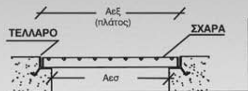
ΤΟΜΗ ΚΑΝΑΛΙΟΥ
