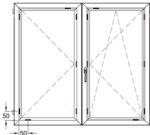
Ανοιγόμενο Opening
