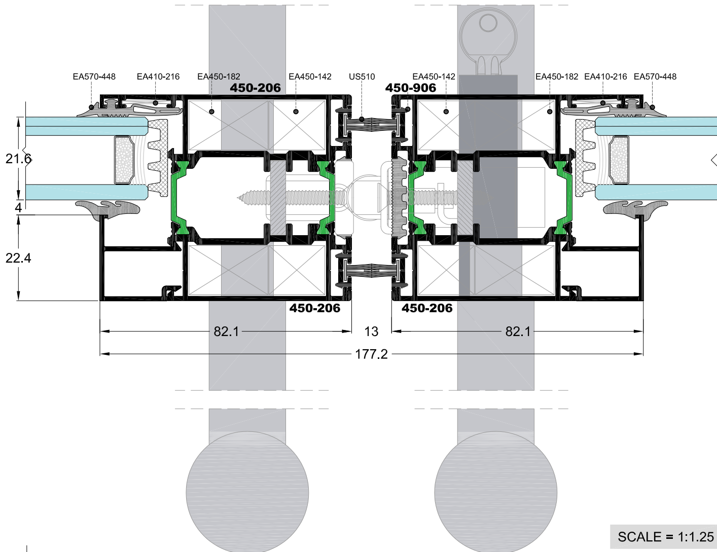
Έξω Πλευρά Outside
