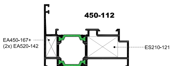
ΓΩΝΙΕΣ ΣΥΝΔΕΣΕΩΣ CORNER JOINT
