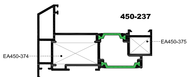
ΓΩΝΙΕΣ ΓΩΝΙΑΣΤΡΑΣ CRIMPING CORNER
