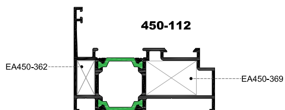
ΓΩΝΙΕΣ ΓΩΝΙΑΣΤΡΑΣ CRIMPING CORNER
