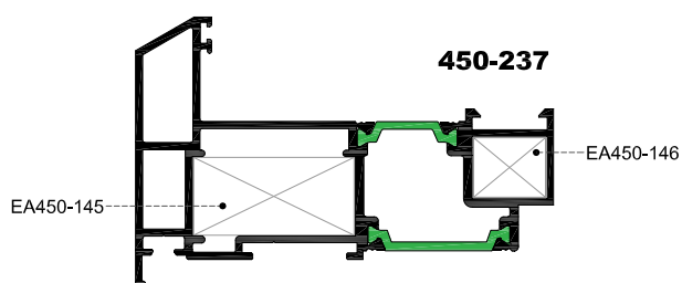
ΓΩΝΙΕΣ ΣΥΝΔΕΣΕΩΣ CORNER JOINT
